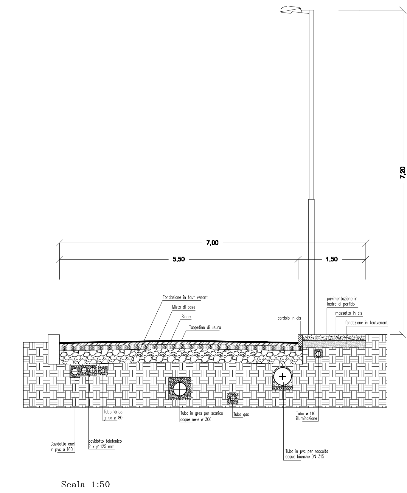
Sezione A - A° Sezione trasversale strada di PRG e sottoservizi
